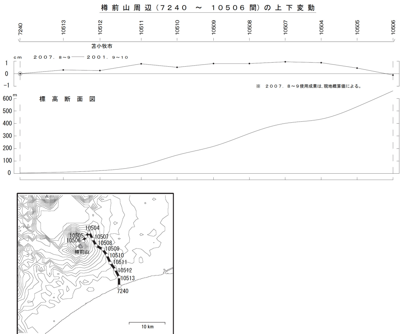
第1図 樽前山周辺の水準測量結果
