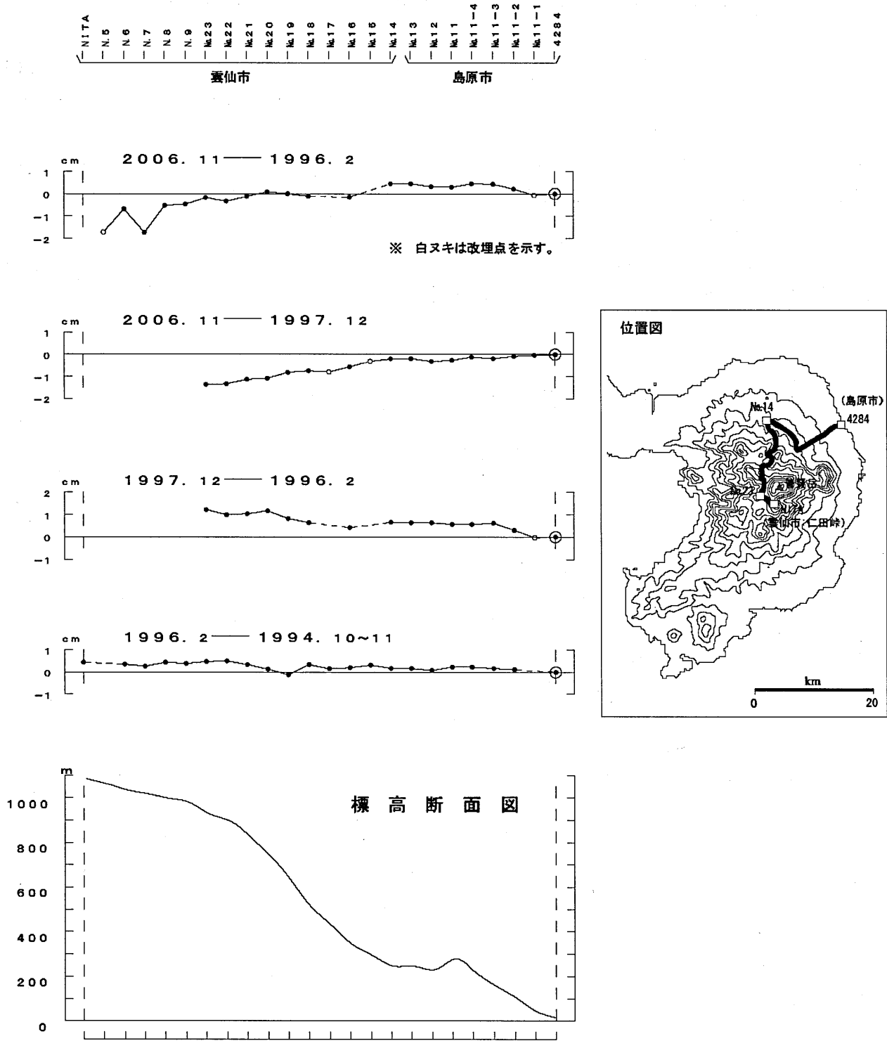
第2図 雲仙岳周辺の水準測量結果
