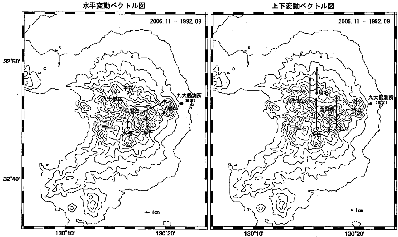
第1図 GPS繰り返し観測から得られた雲仙岳周辺の地殻変動
