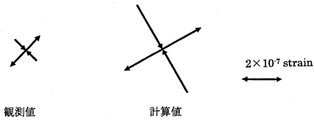
第6図 4月の活動時の歪変化（観測値）と第5図に示す岩脈貫入モデルから求まる歪変化（計算値）。
