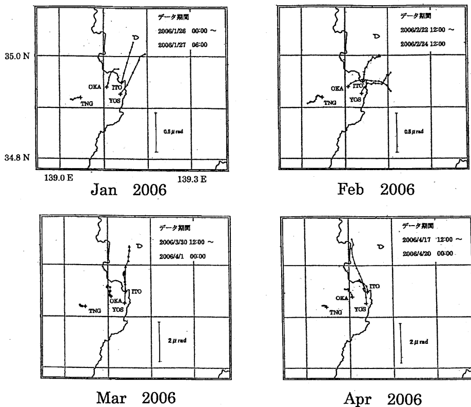
第3図 各時期の傾斜ベクトル
