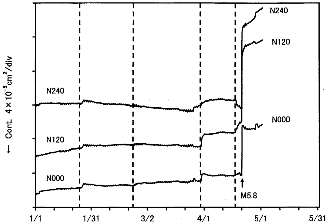
第4図 ITOにおける3成分歪変化. 傾斜と同じように、図中に示す破線より異常な変化が生じ始めている。 Fig.4 Tide removed 3-component strainmeter records at ITO in the period from Jan. 1 to May 1, 2006. Same as the tilt records, broken lines in the figure show the start time of the anomalous strain changes.
