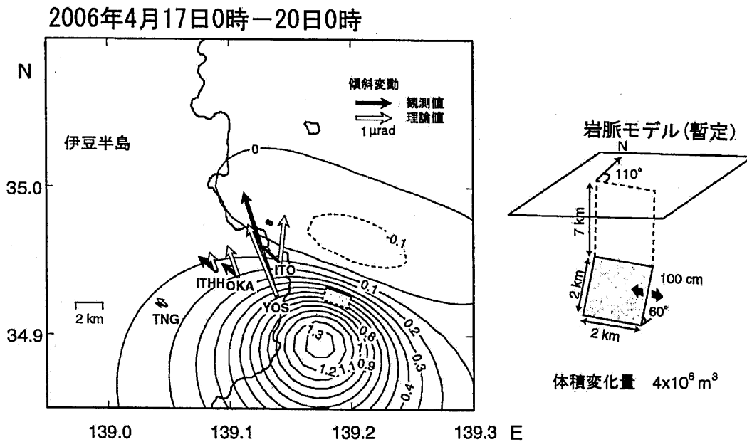
第5図 傾斜観測結果から求めた4月の活動時の岩脈貫入モデル(暫定結果) Fig.5 Dyke intrusion model for the seismo-volcanic activity in April, 2006 inferred from result of tilt observation.
