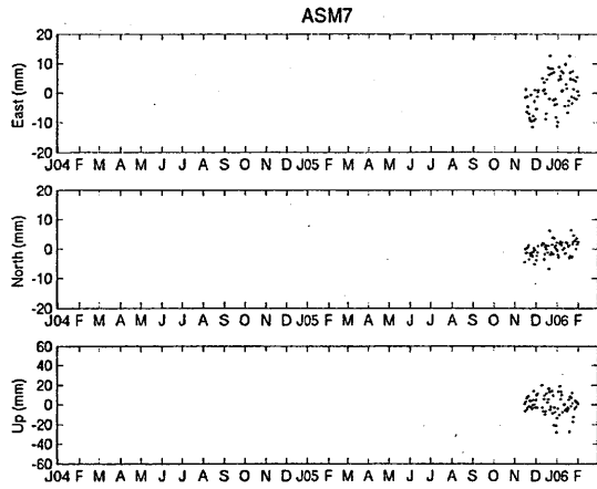
第2図 地震研究所によって連続観測されているGPS観測点の位置変化. 基準点は国土地理院950272観測点である。この点は浅間山から約30 km離れているため不動と考えられる。変動が一番大きいのはASM4であり、噴火前の2004年7月頃から南へ変位し、その変位は2005年中頃まで続いた。ASM4の最近の変動は小さい。2005年1月から2月にかけてのASM6の変動はアンテナ上への積雪の影響と考えられる。
