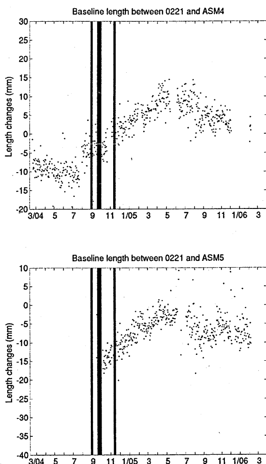
第3図 浅間山を南北に挟む国土地理院950221観測点と東京大学地震研究所ASM4およびASM5観測点の距離変化。太線は中規模噴火の時刻を示す。2004年7月・10月にダイク貫入と思われる山体膨張があり、その後中規模噴火が発生した。2005年1月・4月にもダイク貫入イベントがあったが、噴火には至らなかった。その後、2005年6月頃から山体収縮に転じている。そのレートは2004年7月以前のレートより大きく見えるが、9月以降収縮が止まっているようにも見える。
