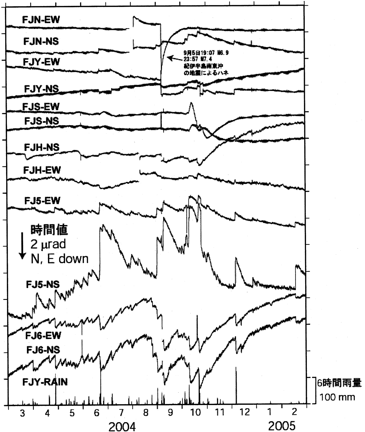
第4図 防災科学技術研究所・富士山火山活動観測網による傾斜変動観測結果。
