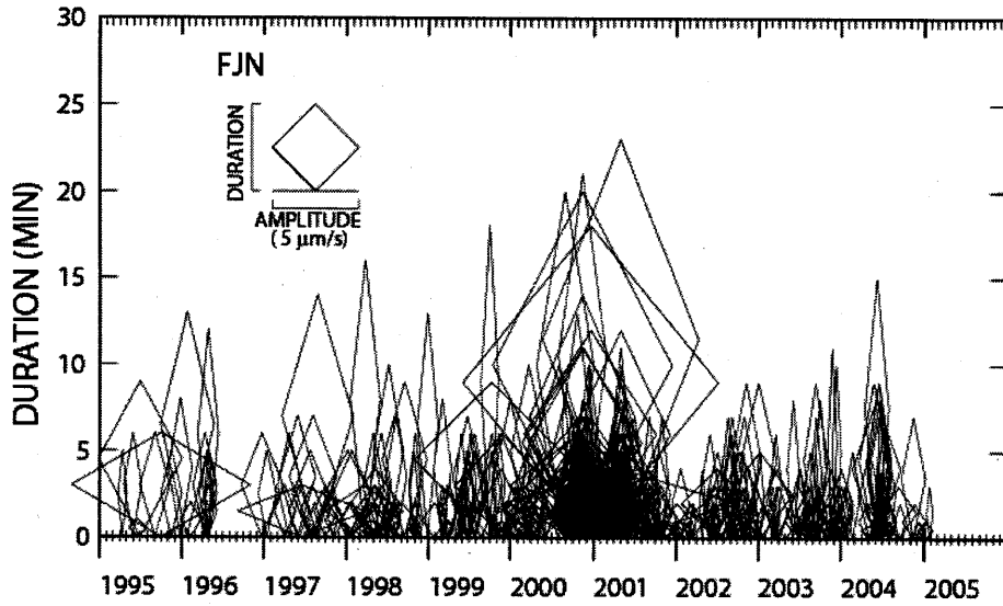
第2図 1995年1月から2005年2月15日までの富士山の低周波地震活動を示す菱形ダイアグラム。 菱形の高さは特定の観測点で観測された低周波地震活動の振動継続時間、幅は最大振幅に対応する。
