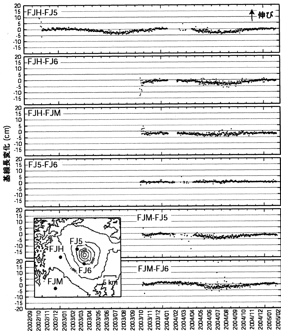
第5図 防災科学技術研究所・富士山火山活動観測網によるGPS観測結果。
