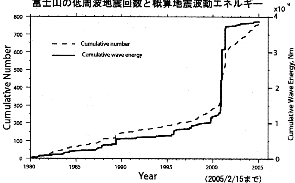
第3図 積算低周波地震回数（破線）と積算概算波動エネルギー（1980年1月1日～2005年2月15日）。 概算波動エネルギーEは、 E=A_{\max}^2 \times TD/T_0 、 A_{\max} とTDは特定観測点での最大振幅と振動継続時間、 T_0 は卓越周期、でここでは一定として扱っている。
