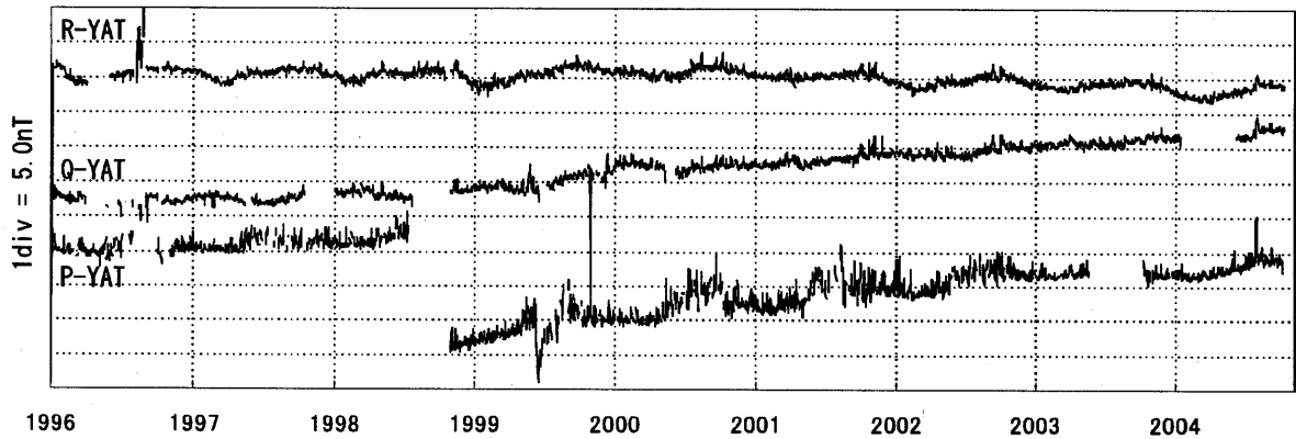
第3図 全磁力連続観測点(P、Q、R)の全磁力変化。
