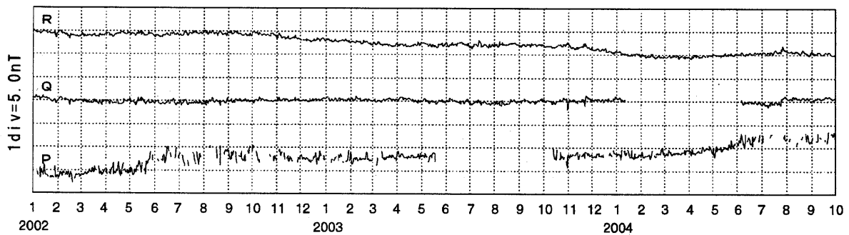
第4図 全磁力連続観測点(P、Q、R)のデータに対して確率差分法を用いた全磁力変動。
