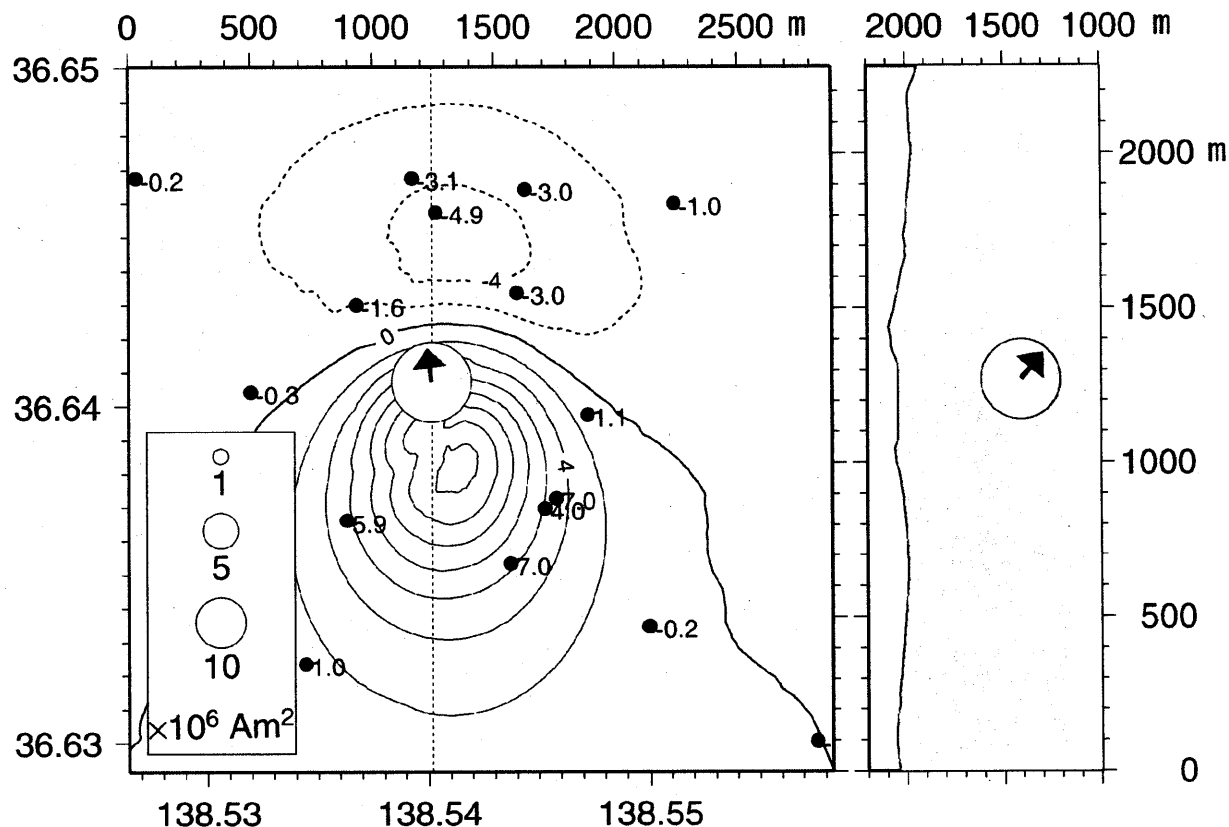
第5図 2000年から2004年までの4年間の全磁力変化量から求めた最適なダイポールの位置と強さ。
