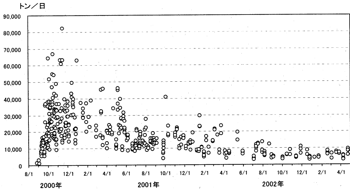
第1図 COSPECによる二酸化硫黄 (SO 2 ) 放出量 (資料期間：2000年9月9日～2003年5月1日) Fig.1 SO 2 emission rate (ton/day) by airborne COSPEC.
