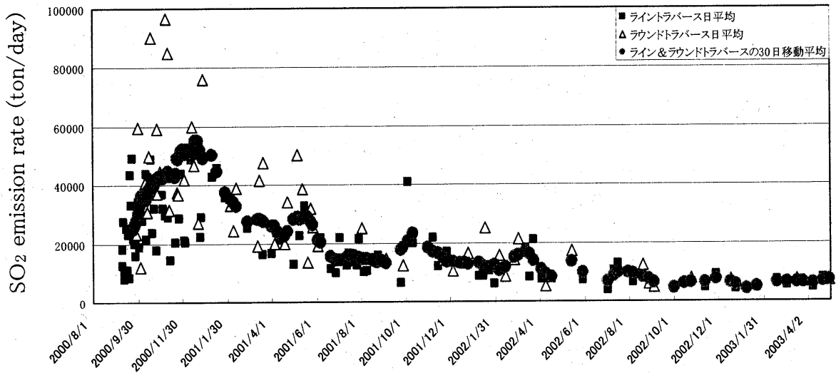
第2図 二酸化硫黄 (SO 2 ) 放出量のトラバース別日平均値と30日移動平均値 (資料期間：2000年9月9日～2003年5月1日) Fig.2 Daily average and moving average of SO 2 flux obtained by airborne COSPEC. Square : daily average by line-traverse observation. Triangle: daily average by round-traverse observation. Circle : 30 days moving average of both observations.
