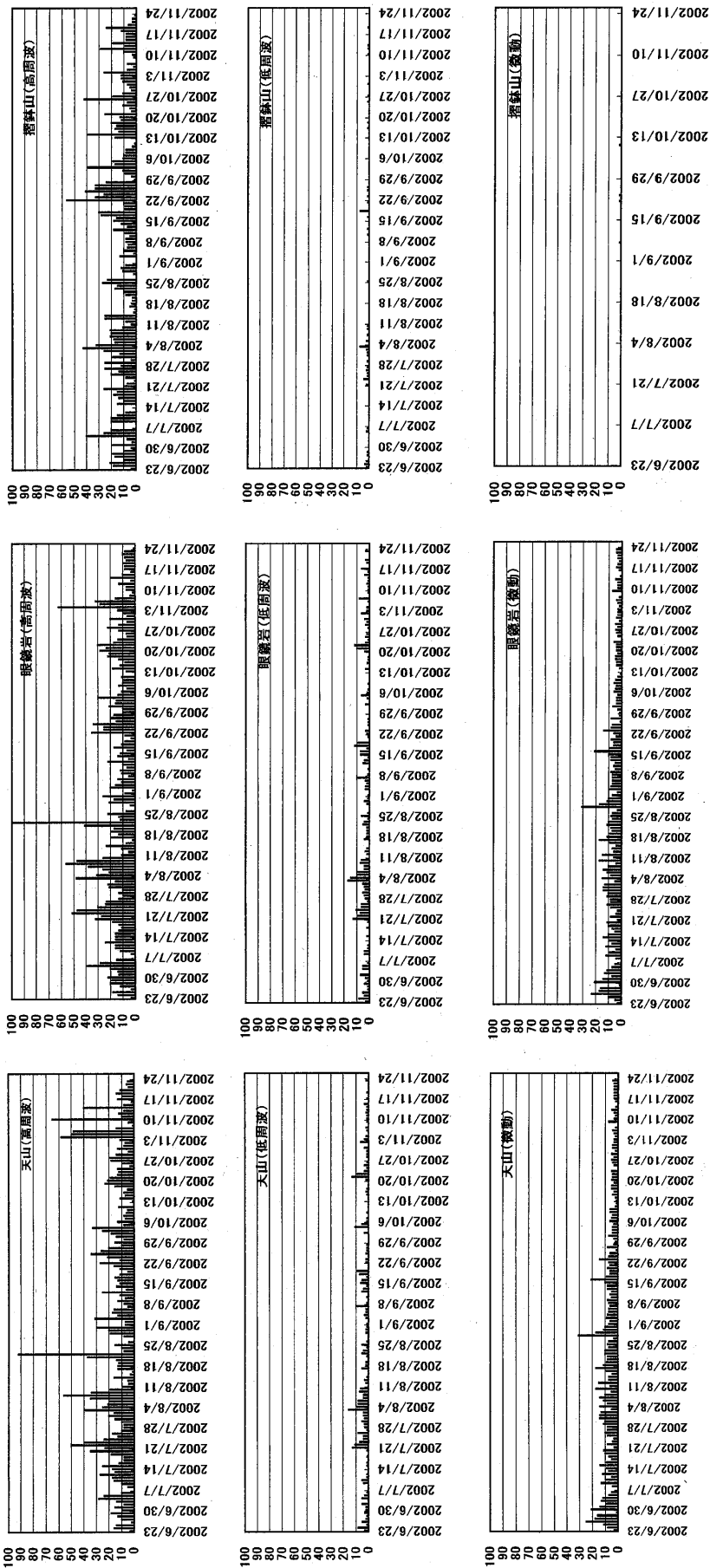
第2図 硫黄島で発生する高周波地震,低周波地震および火山性微動の日別発生回数 Fig.2 Daily numbers of HF, LF earthquakes and volcanic tremor at Iwojima volcano.
