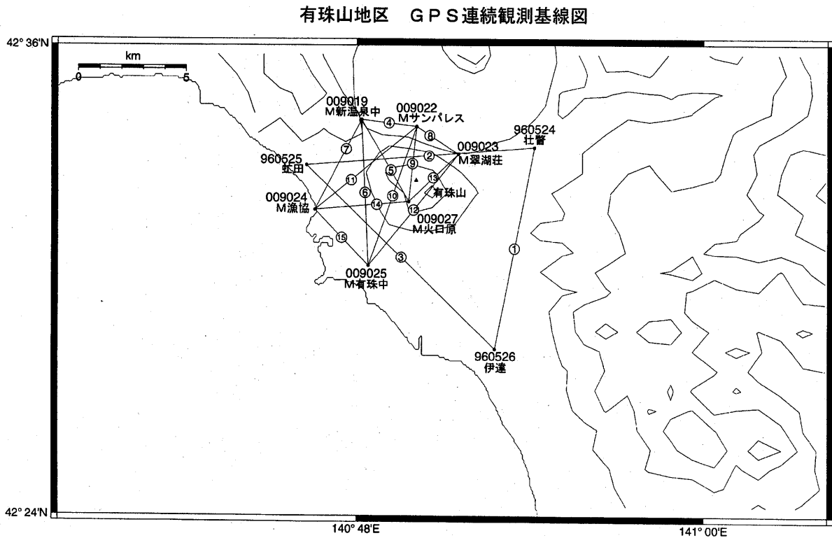
第1-1図 有珠山周辺のGPS連続観測結果(2000年3月～2002年10月)
