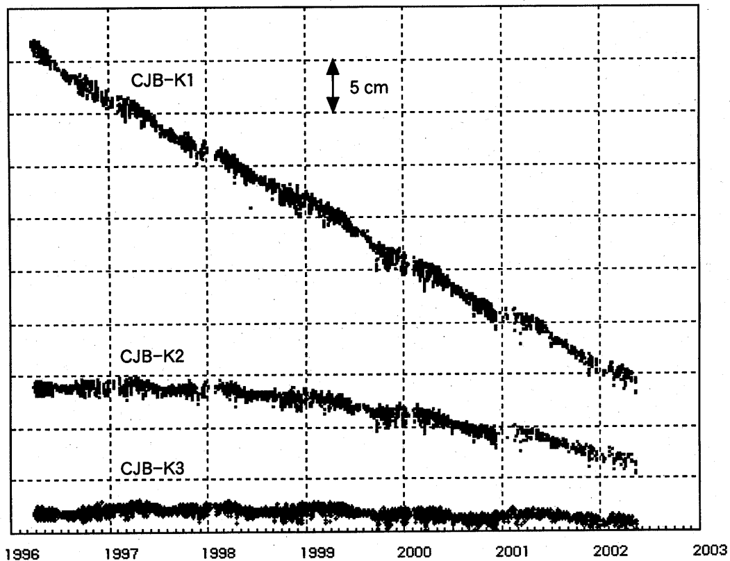
第2図 長者原-K1~K3間の斜距離変化
