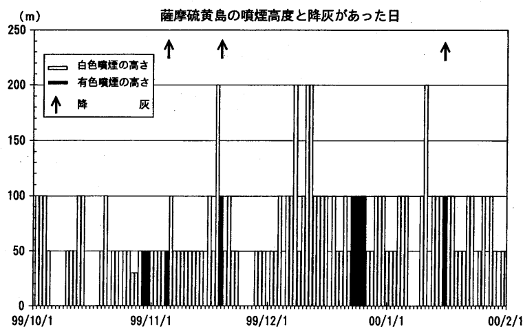
第2図 日別噴煙高度（1999年10月1日～2000年1月31日：三島村役場硫黄島出張所による） Fig. 2 Daily height of volcanic plume. (Oct. 1 1999—Jan. 31 2000)
