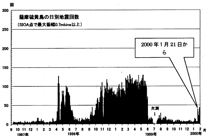
第1図 薩摩硫黄島の日別地震回数（1997年9月10日～2000年1月31日） Fig. 1 Daily frequency of volcanic earthquakes at Satsuma-Iojima volcano. (Sep. 10 1997—Jan. 31 2000)
