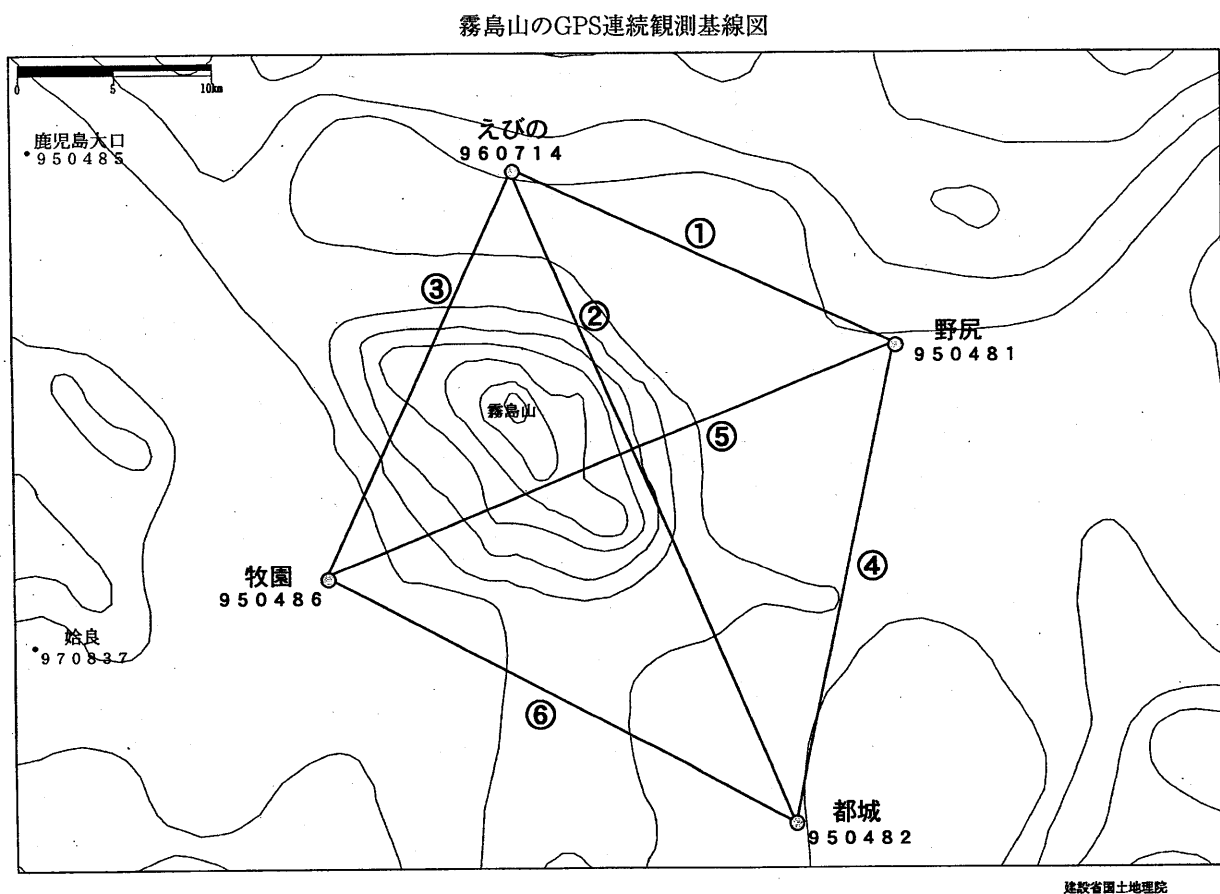
第1-1図 霧島山周辺のGPS連続観測基線図
