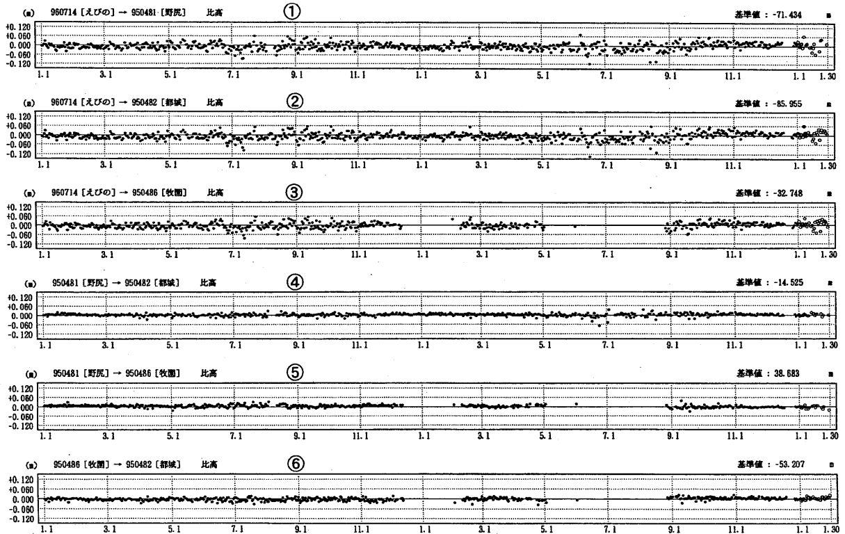
第1-2図 霧島山周辺におけるGPS連続観測結果：1998年1月～2000年1月
