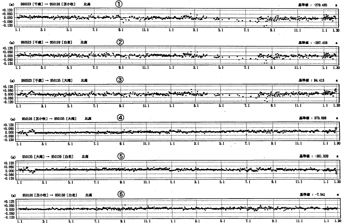
第1-2図 樽前山周辺におけるGPS連続観測結果：1998年1月~2000年1月
