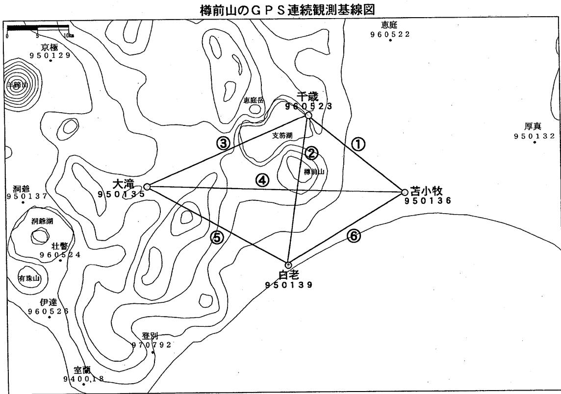
第1-1図 樽前山周辺のGPS連続観測基線図
