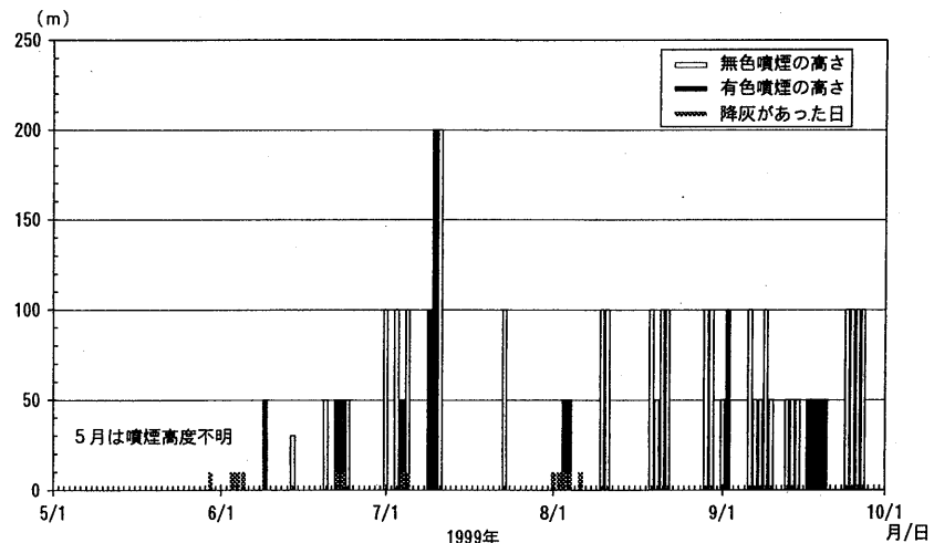
第2図 日別噴煙高度(1999年5月1日～9月30日;三島村役場硫黄島出張所による) Fig.2 Daily height of volcanic plume. (May 1—Sep. 30 1999)
