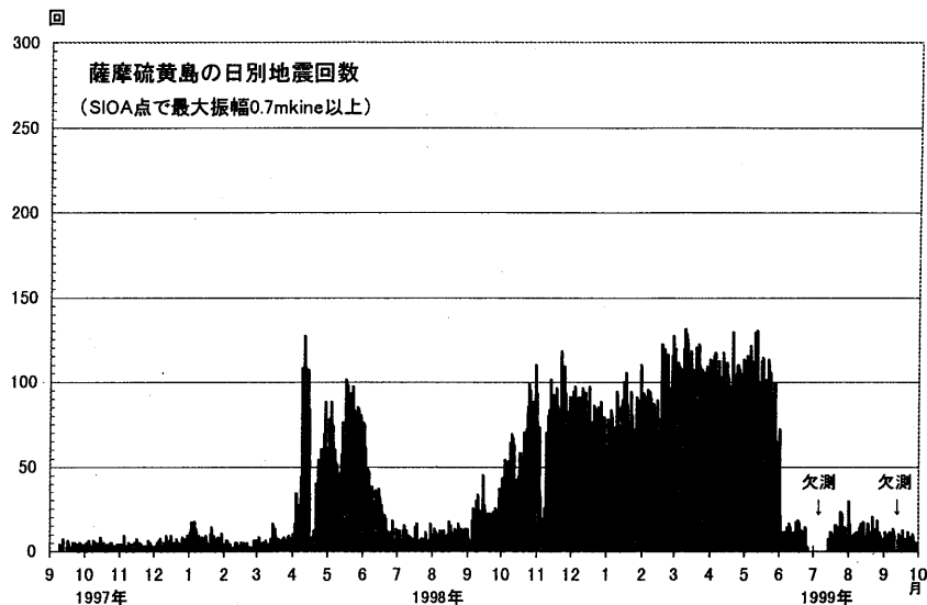
第1図 薩摩硫黄島の日別地震回数(1997年9月10日～1999年9月30日) Fig.1 Daily frequency of volcanic earthquakes at Satsuma-Iojima volcano. (Sep. 10 1997—Sep. 30 1999)
