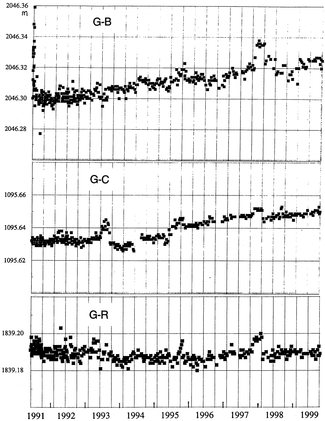
第2図 眉山東斜面の光波測距観測結果
