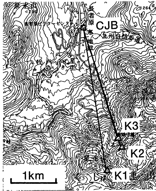
第1図 九重火山光波測距観光網。K1, K2, K3は反射鏡, CJBは器械点。 Fig.1 EDM network on Kuju volcano. K1 to K3 : targets, and CJB : instrument station.
