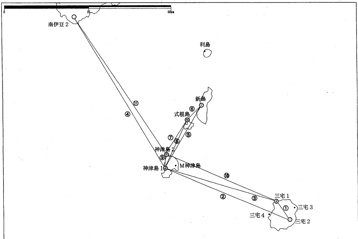
第1-1図 神津島周辺のGPS連続観測点配置と基線
