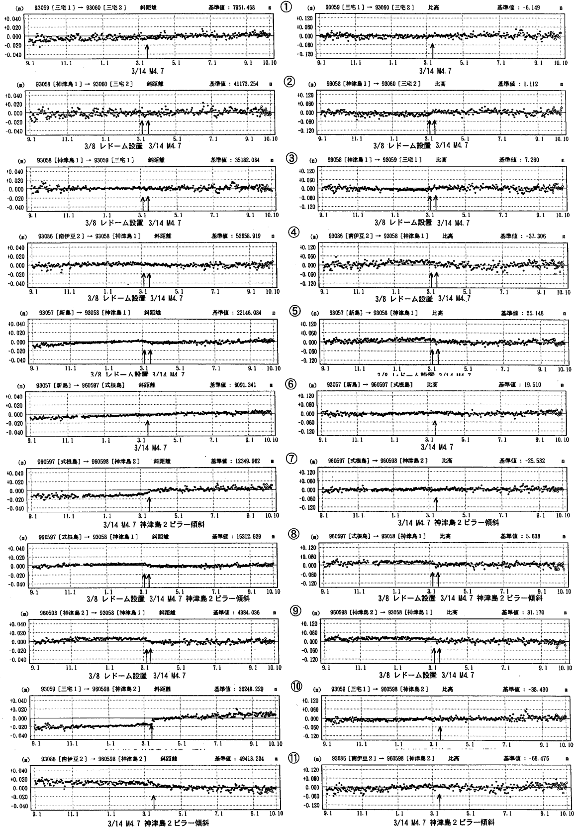
第1-2図 神津島周辺の各GPS観測点間の基線長変化1998年9月-1999年10月
