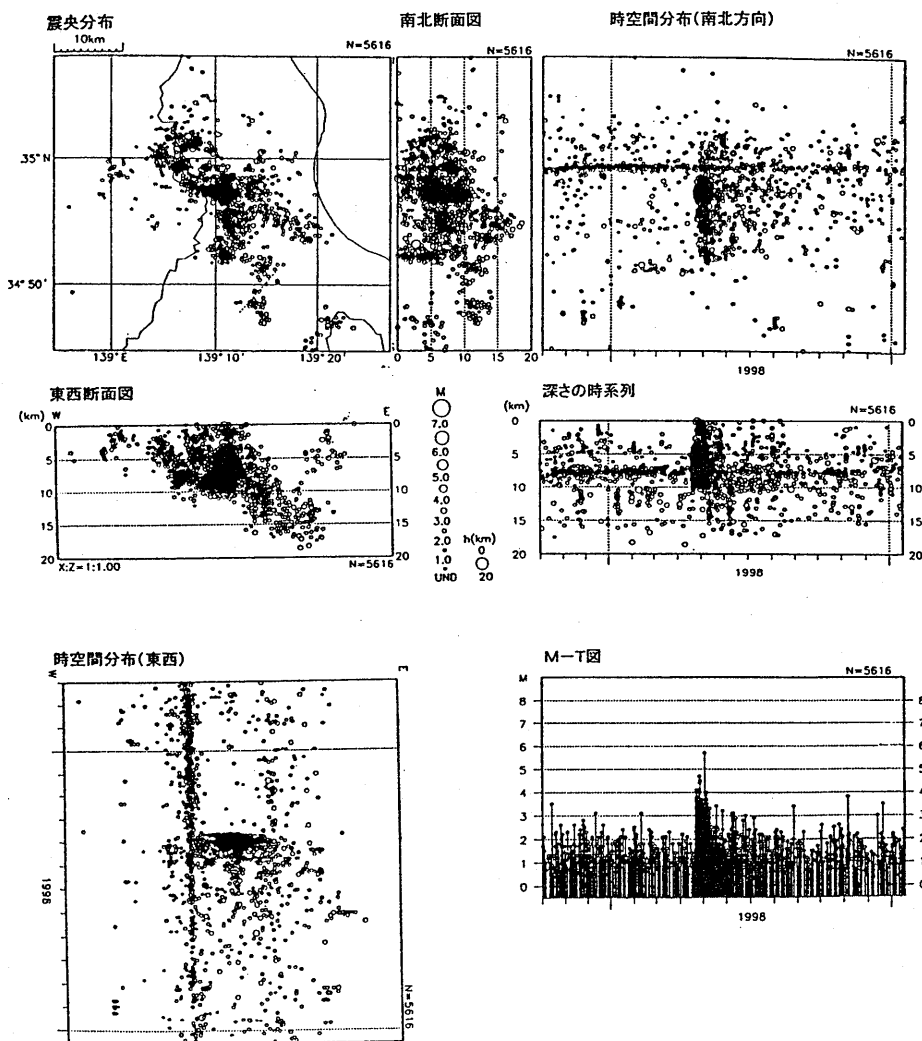
第1図 伊豆半島東方の地震活動（1997年10月1日～1999年1月17日）
