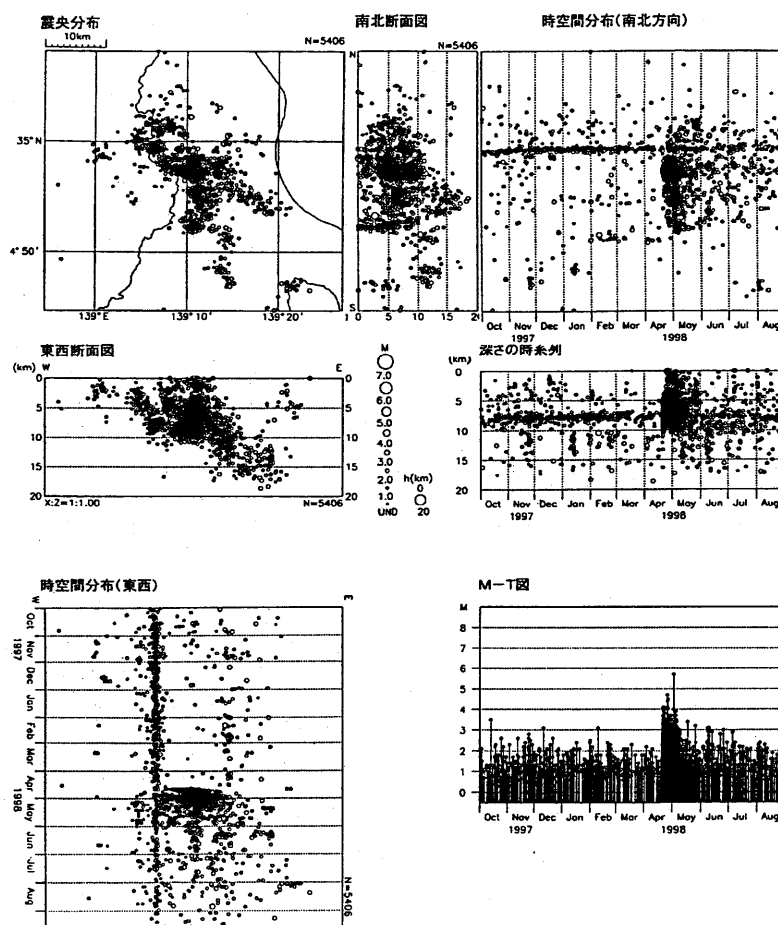
第1図 伊豆半島東方の地震活動。(1997年10月1日～1998年9月19日)
