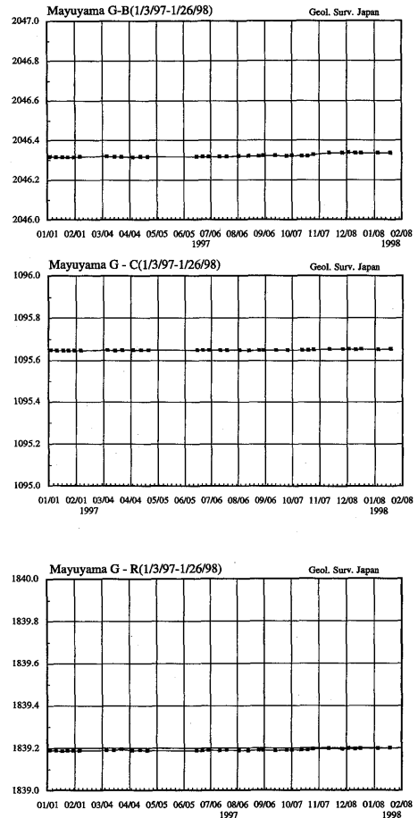
第2図 G-B、G-C及びG-R測線の斜距離変化 Fig.2 Changes in slope distance of Mayu-yama network, G-B, G-C and G-R.
