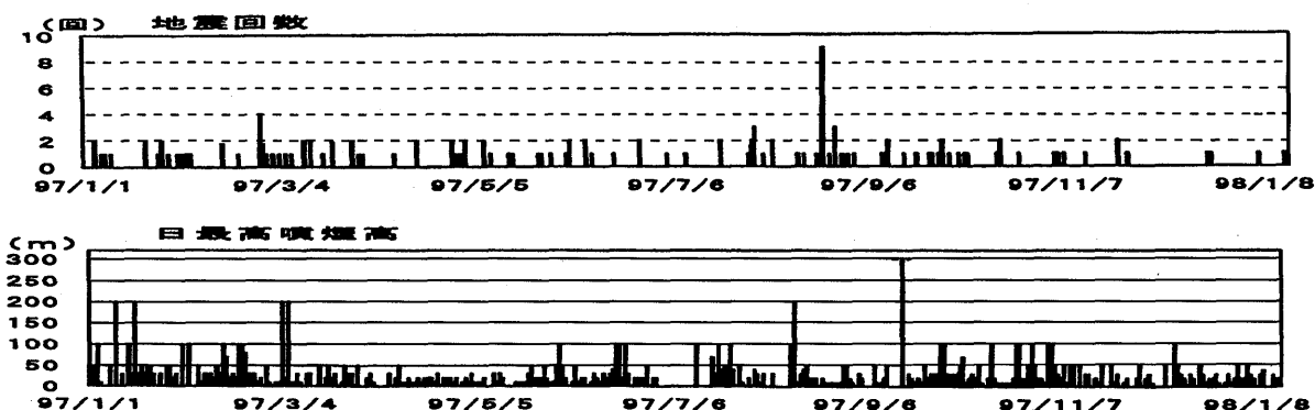
第1図 雲仙岳日別グラフ (1997年1月1日~1998年1月8日)
