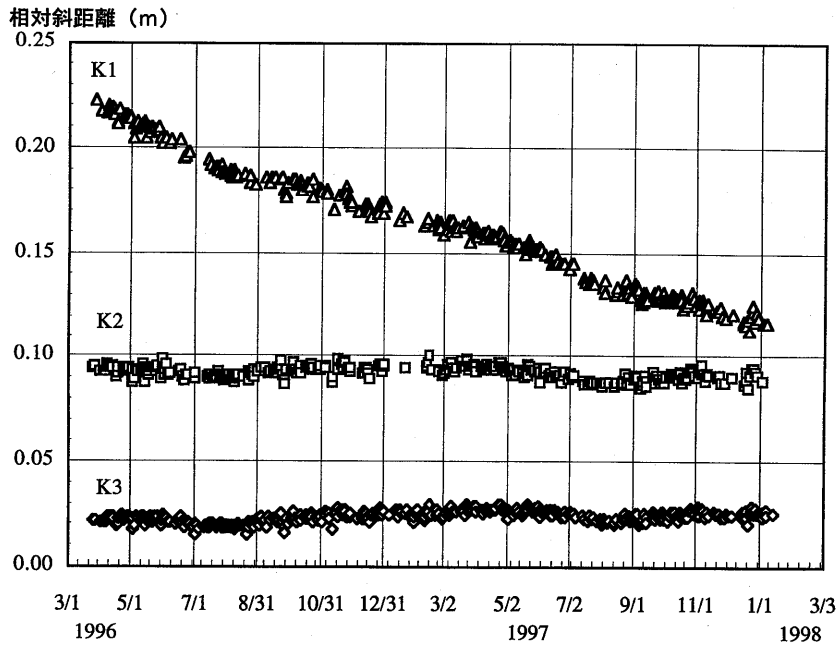
第2図 長者原-K1-3間の斜距離変化。自動連続光波測距による。日没前約2時間のデータを選択し、その平均をそれぞれ3244.70、2782.95、2529.45mシフトさせて表示した。 Fig.2 Change in slope distances between Chojabaru and K1 to K3 using automatic EDM system. Selected data in the stable atmospheric condition in the evening are plotted. Add 3244.70, 2782.95, and 2529.45m for each line.
