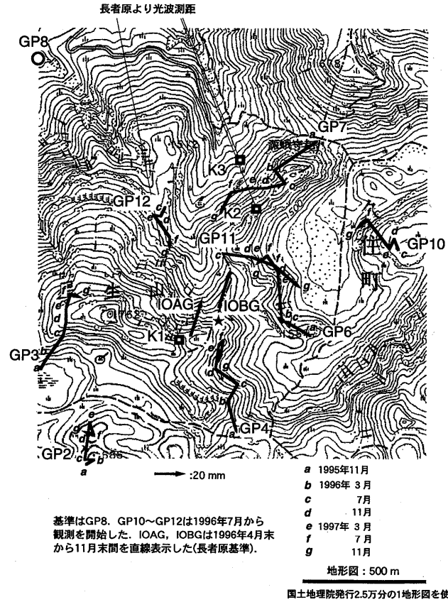
第1図 九重火山山体変動観測. K1、K2、K3は光波測距用反射鏡、GP2-12、IOAG、IOBG、GPS観測点、矢印は1995年11月から1997年11月までのGPS観測による水平変動ベクトル。 Fig.1 Ground deformation measurement network on Kuju volcano. K1 to K3:targets for EDM, IOAG and IOBG:automatic GPS station, arrow:horizontal movement vector by GPS measurement, between November 1995 and November 1997.
