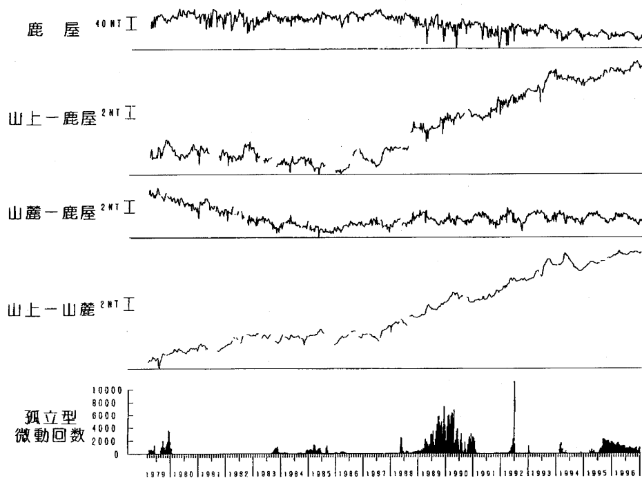
第2図 地磁気全磁力夜間値の相互差（阿蘇山上－鹿屋、阿蘇山麓－鹿屋、阿蘇山上－阿蘇山麓）の旬平均値変化。これら3つとも鹿屋のH成分を用いて、地磁気の外部磁場擾乱の補正を施してある。（阿蘇山上－阿蘇山麓）はその他に年周変化の補正も施してある。最下段は孤立型微動の旬回数。（1979年3月～1996年12月）
