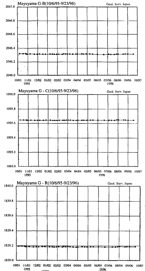
第2図 G-B, G-C及びG-R測線の斜距離変化 Fig.2 Changes in slope distances of Mayu-yama network, G-B, G-C and G-R.
