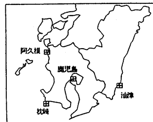
第1図 鹿児島島・阿久根・枕崎・油津各験潮場間の月平均潮位差 Fig. 1 Differences in monthly mean sea level between Kagoshima, Akune, Makurazaki and Aburatsu tidal stations.
