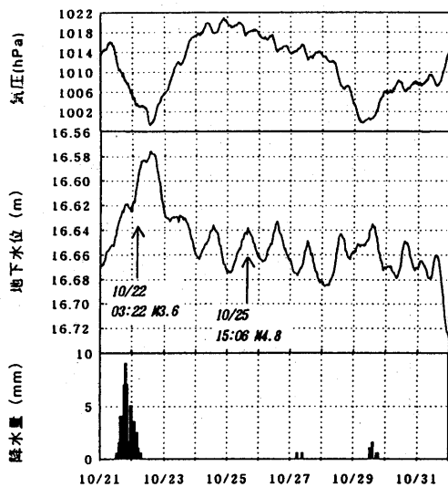
第 8 図 大井観測井の地下水位記録。左は10月21日から31日、右は10月25日0時から24時まで。 Fig. 8 Change in groundwater level in the Ooi observation well. (Left) Oct. 21 - Oct. 31, 1994. (Right) Oct. 25, 1994.
