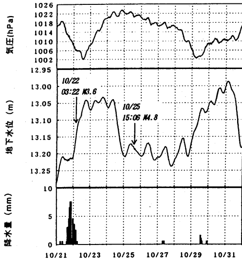
第 9 図 小田原観測井の地下水位記録。左は10月21日から31日，右は10月25日0時から24時まで。
