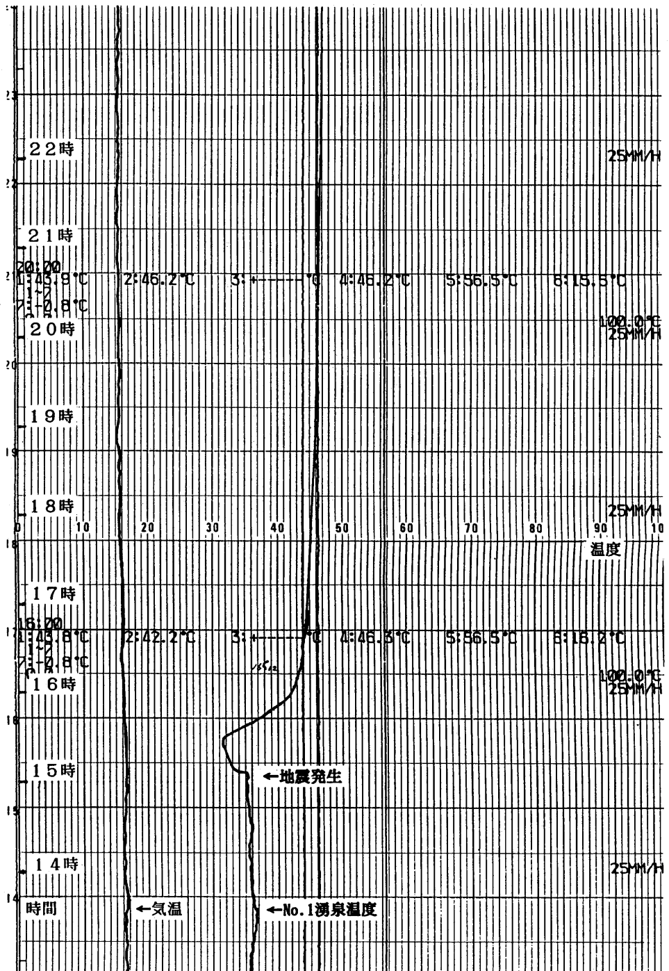
第 6 図 箱根湯本第 3 号源泉の温度記録
