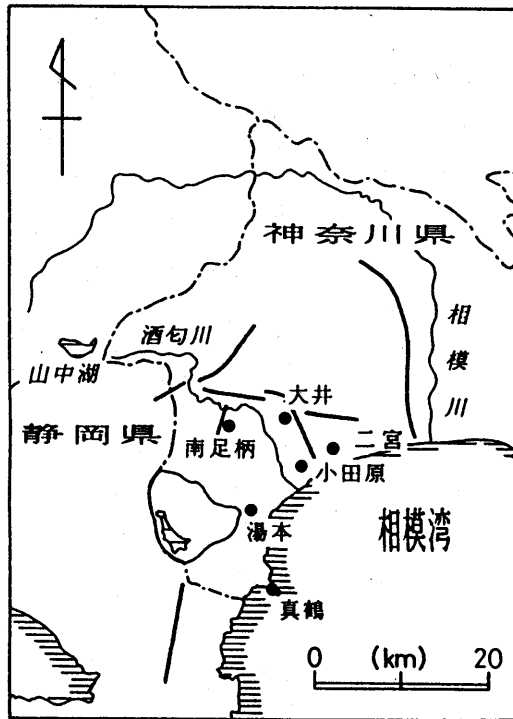
第 7 図 地下水位観測井の位置 Fig. 7 Location of groundwater level observation wells.
