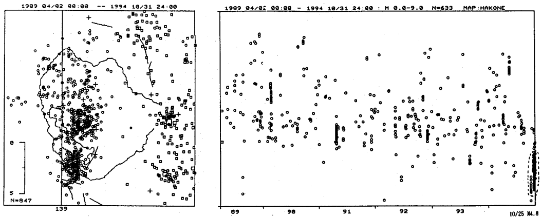
第4図 箱根火山周辺地域の震央分布と時空間分布（1989年4月～1994年10月まで） Fig. 4 (Left) Epicentral distribution of earthquakes. (Right) Space-time distribution of earthquakes in the Hakone volcano and adjacent areas (April, 1989–October, 1994).
