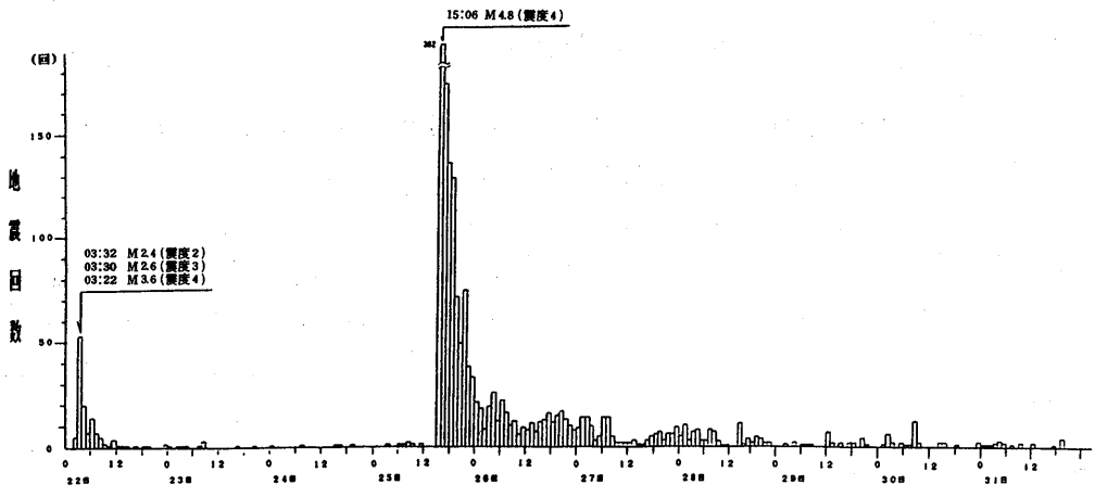
第 1 図 箱根・駒ヶ岳観測点における時間別頻度分布 (1994年10月22日～10月31日) Fig. 1 Hourly frequency of earthquakes at Hakone・Komagatake (October 22 -October 31, 1994).
