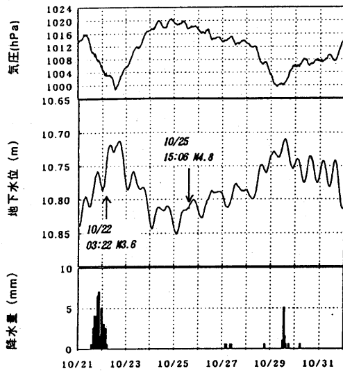
第 10 図 二宮観測井の地下水位記録。左は10月21日から31日，右は10月25日0時から24時まで。
