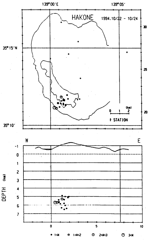
第 2 図 震源分布 (10月22日～10月24日) Fig. 2 Hypocenter distribution (October 22-October 24, 1994).
