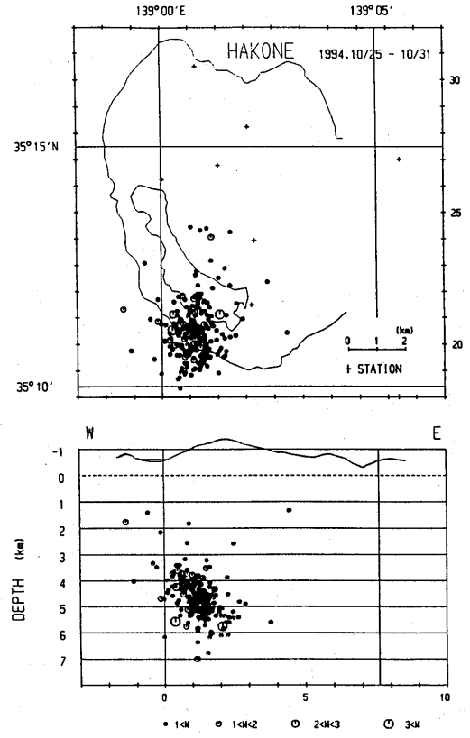
第 3 図 震源分布 (10月25日～10月31日) Fig. 3 Hypocenter distribution (October 25 -October 31, 1994).
