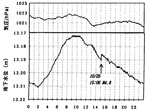
小田原観測井 941025
