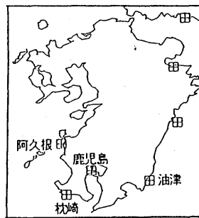
第1図 鹿兒島・阿久根・枕崎・油津各験潮場間の月平均潮位差
