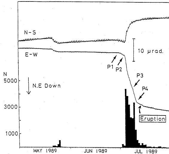
第4図 伊東観測点における傾斜記録と気象庁の鎌田における日別地震回数 (1989年5月1日から7月31日まで)
