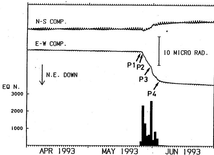
第2図 伊東観測点における傾斜記録と気象庁の鎌田における日別地震回数（1993年4月1日から6月30日まで）
