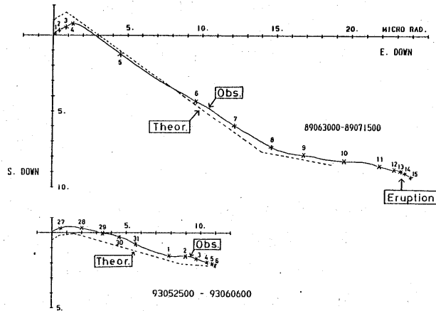
第6図 第5図に示すモデルの結果(破線)と観測値(実線)との比較。上段は1989年, 下段は1993年の活動時を示す。
