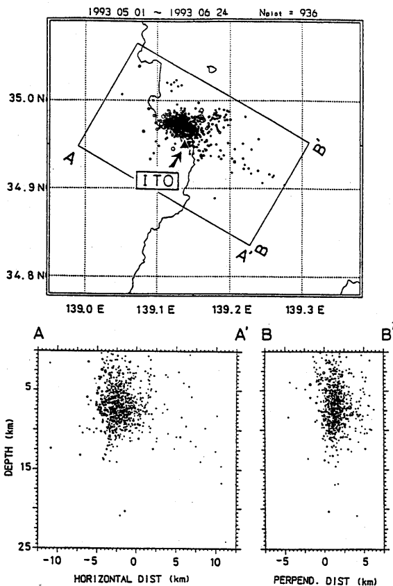
第1図 1993年の群発地震の震源分布。伊東観測点の位置を▲で示す。
