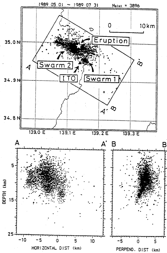
第3図 1989年の群発地震の震源分布
