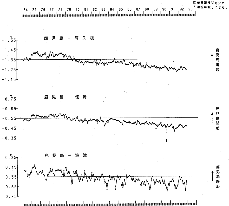
第1図 鹿児島・阿久根・枕崎・油津各験潮場間の月平均潮位差
