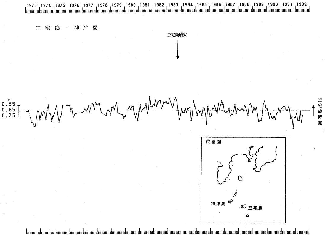
第1図 三宅島・神津島験潮場間の月平均潮位差
