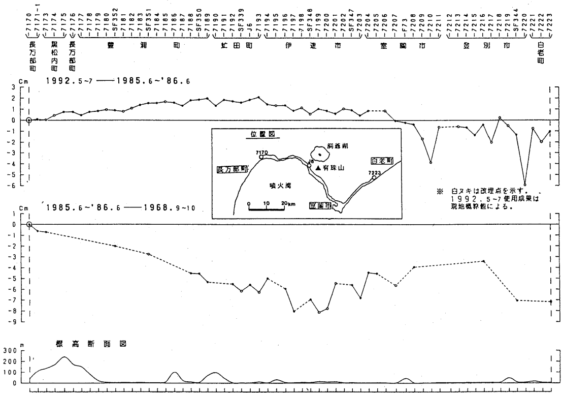
第1図 長万部～白老間の上下変動
