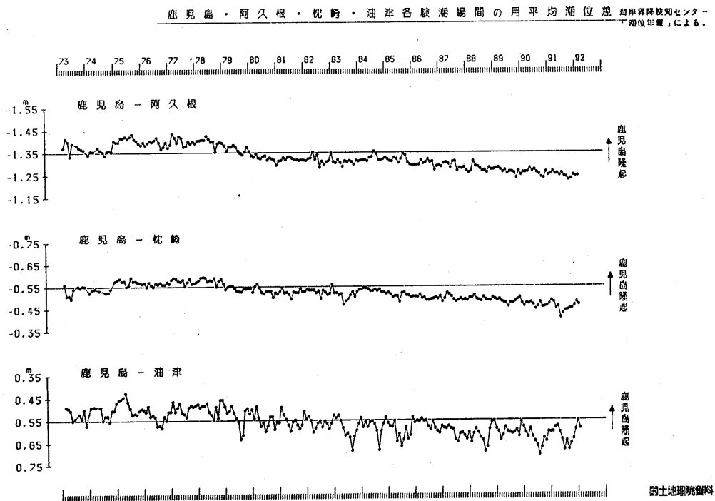
第1図 鹿児島・阿久根・枕崎・油津各験潮場間の月平均潮位差
