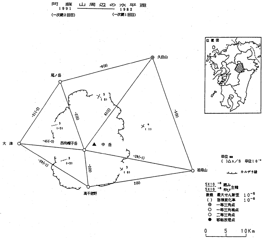
第1図 阿蘇山周辺の水平歪
