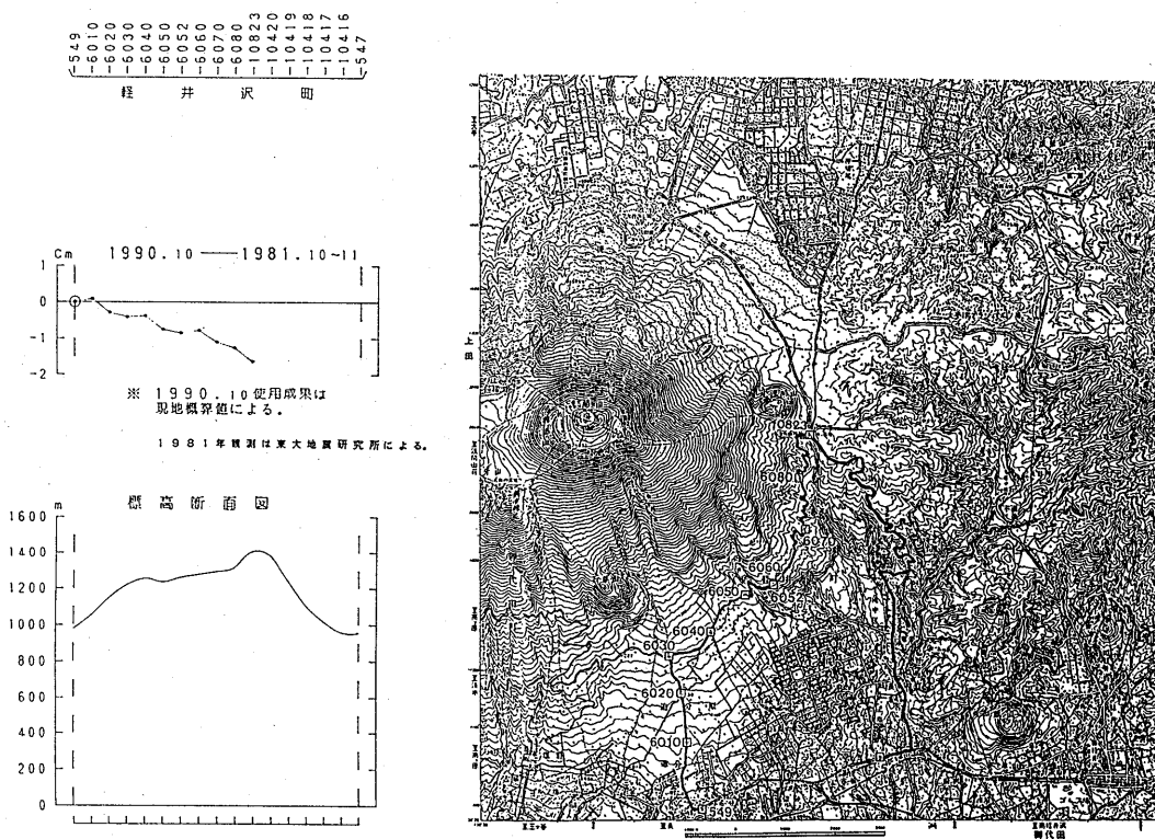
第1図 浅間山水準路線図(右)と水準測量結果(左)
