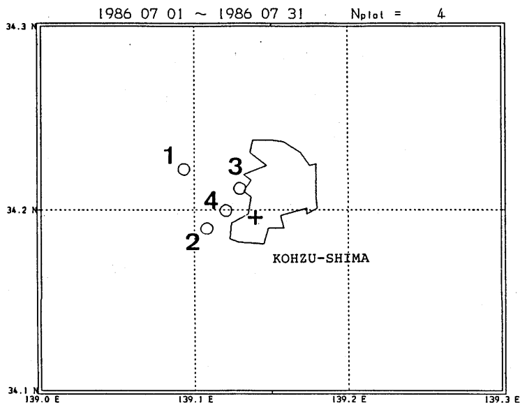
第1図 神津島付近の1986年7月の震央分布（数字は本文中の地震番号に対応）
