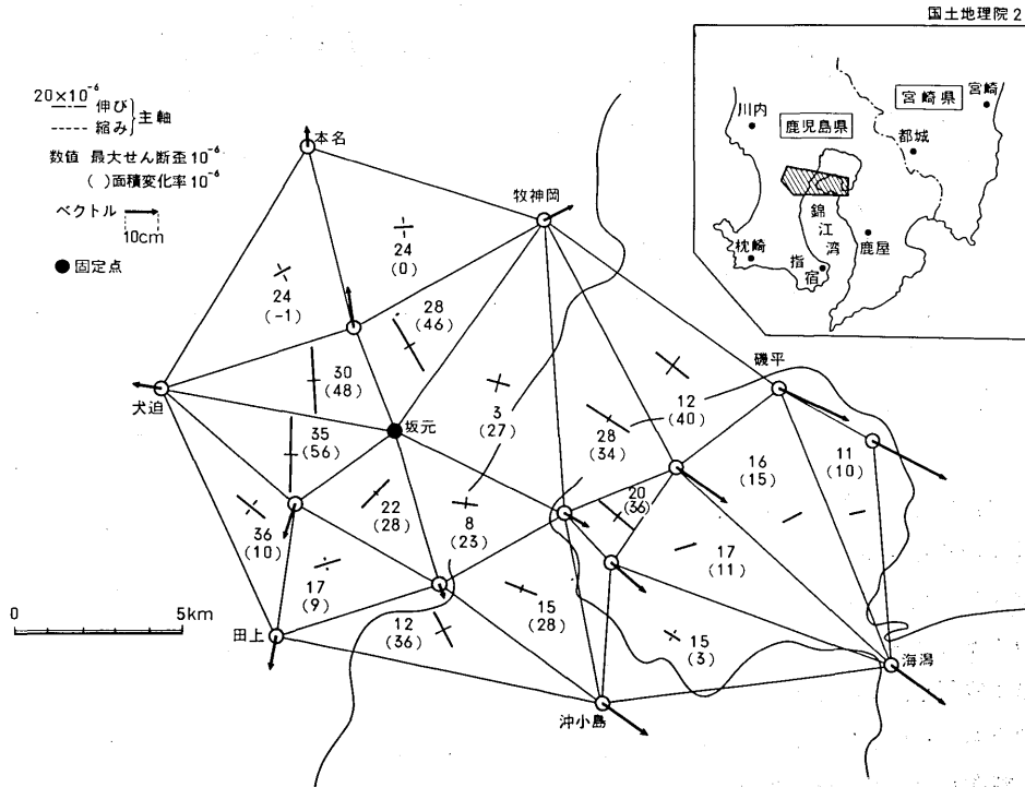
第1図 桜島付近の水平変動(1977-1970)
