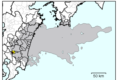
噴火開始から14時までの降灰量
