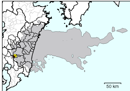
噴火開始から10時までの降灰量
