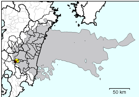
噴火開始から09時までの降灰量
