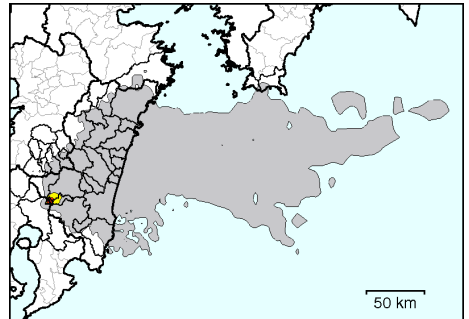
噴火開始から11時までの降灰量
