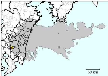
噴火開始から12時までの降灰量
