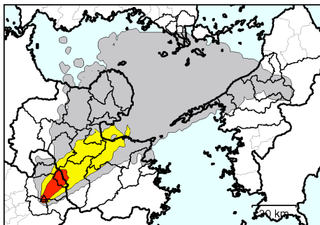
噴火開始から05時までの降灰量
