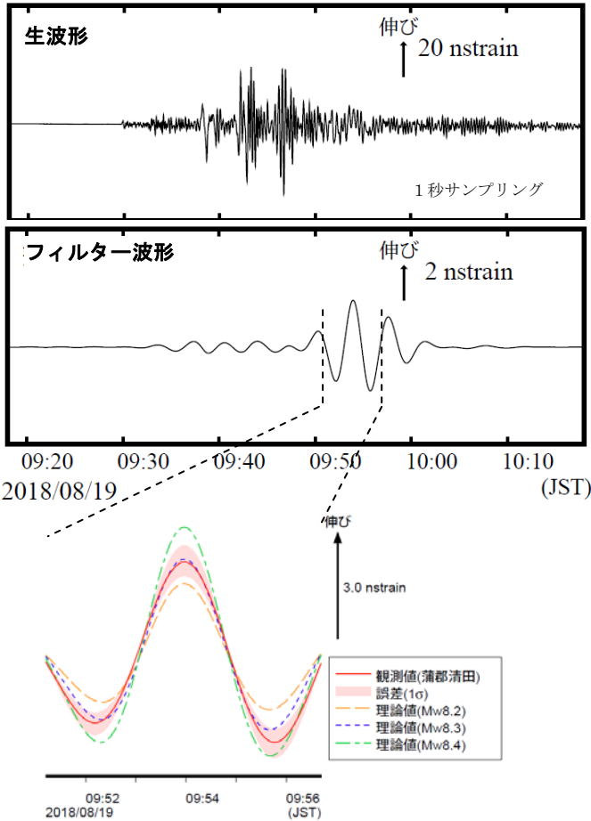
蒲郡清田観測点の観測波形と理論波形の振幅比較 (上図) データには周期 180-333 秒のバンドパスフィルタを時間軸の正逆両方向にかけている。網掛けは誤差 ( 1\sigma ) の範囲を示す。
