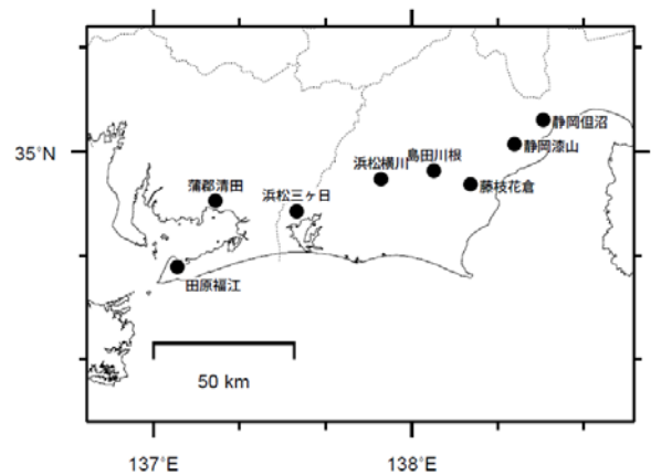
理論波形と体積ひずみ観測点 8 カ所の観測波形との比較 (下図) データには周期 180-333 秒のバンドパスフィルタを時間軸の正逆両方向にかけている。
