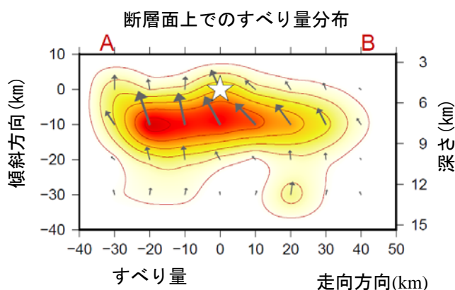
小さい ← → 大きい 星印は破壊開始点、矢印は下盤側に対する上盤側の動きを表す。
