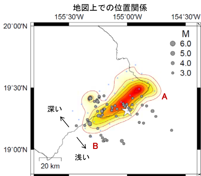
星印は破壊開始点を示す。また、灰色の丸は本震発生後3日以内の地震の震央を示す（ M_{3.0} 以上、USGSによる）。
