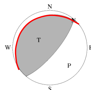
断層面の設定に用いた節面（走向234°、傾斜15°、すべり角103°）を赤線で示す。
