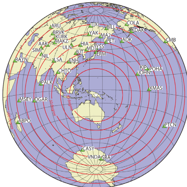
観測点分布
