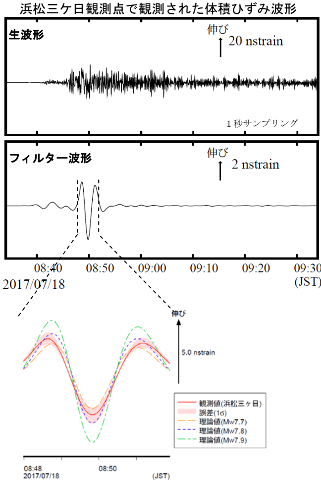
浜松三ヶ日観測点の観測波形と理論波形の振幅比較 (上図) データには周期 120-333 秒のバンドパスフィルタを時間軸の正逆両方向にかけている。網掛けは誤差 (1σ) の範囲を示す。
