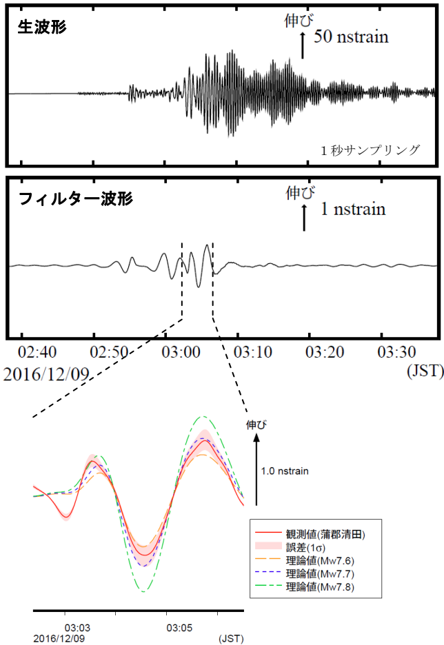
蒲郡清田観測点の観測波形と理論波形の振幅比較 (上図) データには周期 120-333 秒のバンドパスフィルタを時間軸の正逆両方向にかけている。網掛は誤差 (1 \sigma ) の範囲を示す。
