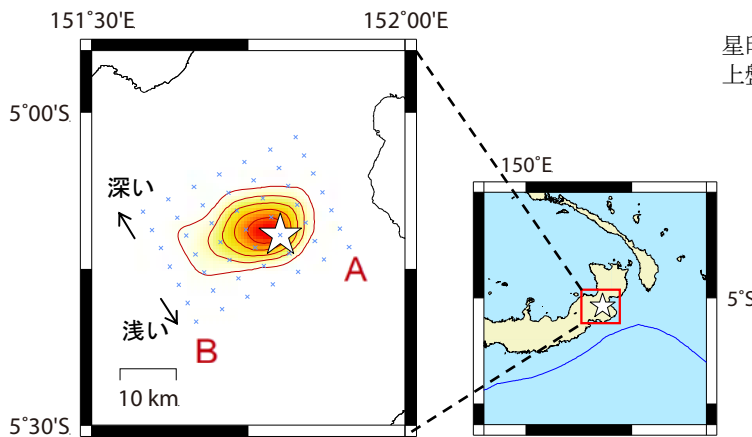
星印は初期破壊開始点を示し、青線はプレート境界を示す。
