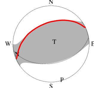
断層面の設定に用いた節面 (走向244°、傾斜44°、すべり角78°) を赤線で示す。
