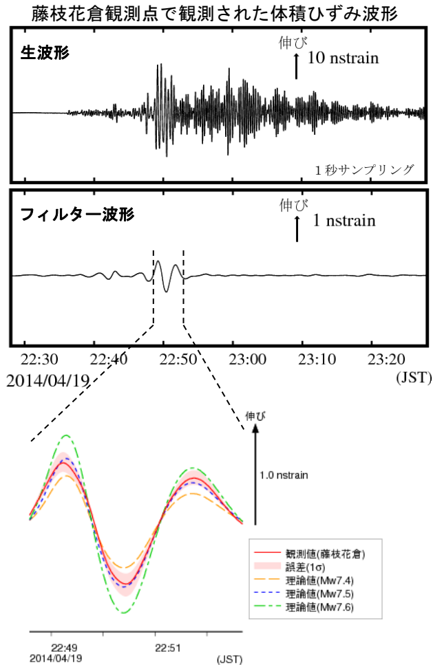
藤枝花倉観測点の観測波形と理論波形の振幅比較（上図） データには周期 120-333 秒のバンドパスフィルタを時間軸の正逆両方向にかけている。網掛けは誤差（1σ）の範囲を示す。
