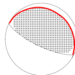
解析に用いたメカニズム解 (気象庁W-phase解)
