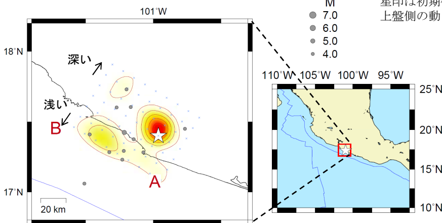
地図上に投影したすべり量分布
