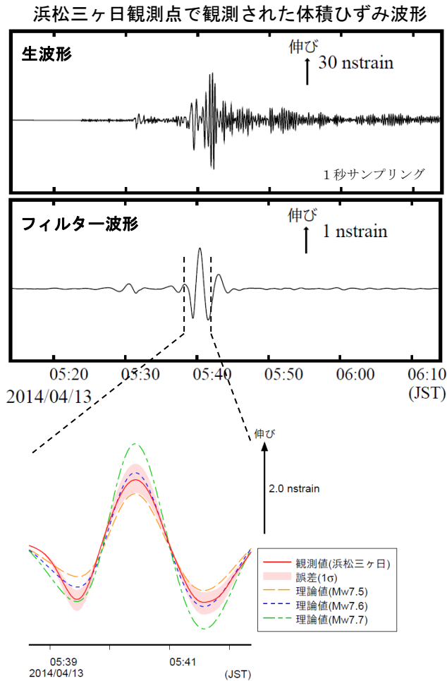
浜松三ヶ日観測点の観測波形と理論波形の振幅比較（上図） データには周期 120-333 秒のバンドパスフィルタを時間軸の正逆両方向にかけている。網掛けは誤差（1 \sigma ）の範囲を示す。
