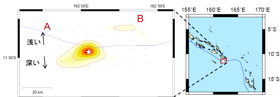
地図上に投影したすべり量分布
