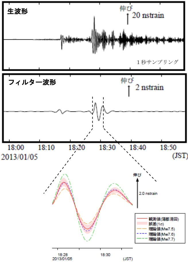
蒲郡清田観測点の観測波形と理論波形の振幅比較 (上図) データには周期 120-333 秒のバンドパスフィルタを時間軸の正逆両方向にかけている。網掛は誤差 (1σ) の範囲を示す。
