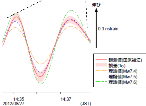
田原福江観測点の観測波形と理論波形の振幅比較（上図） データには周期 120～333 秒のバンドパスフィルタを時間軸の正逆両方向にかけている。網掛けは誤差（1 \sigma ）の範囲を示す。
